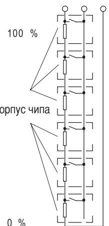
Внутренняя схема датчика уровня
